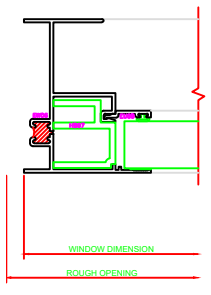
402 JAMB SERIES: 3500
